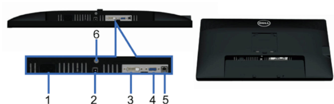
Вид снизу
